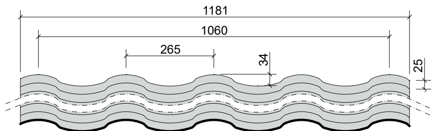
A-A Section
