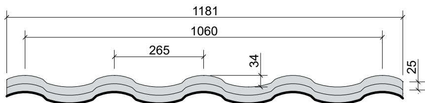
A-A Section
