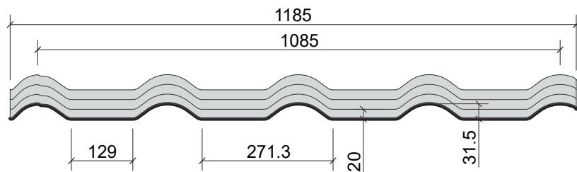
A-A Section
