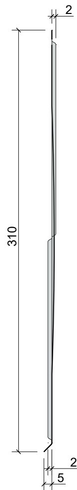
Secțiune B-B
