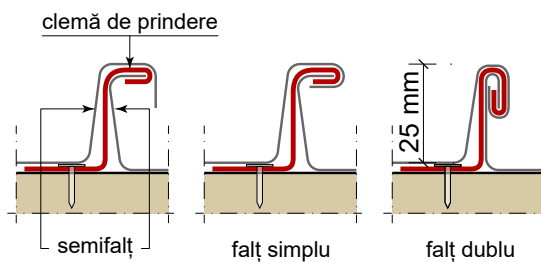
Detalii îmbinare
