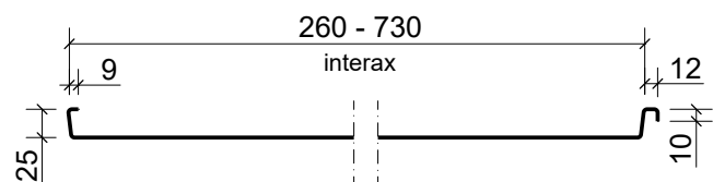
Sețiune A-A
